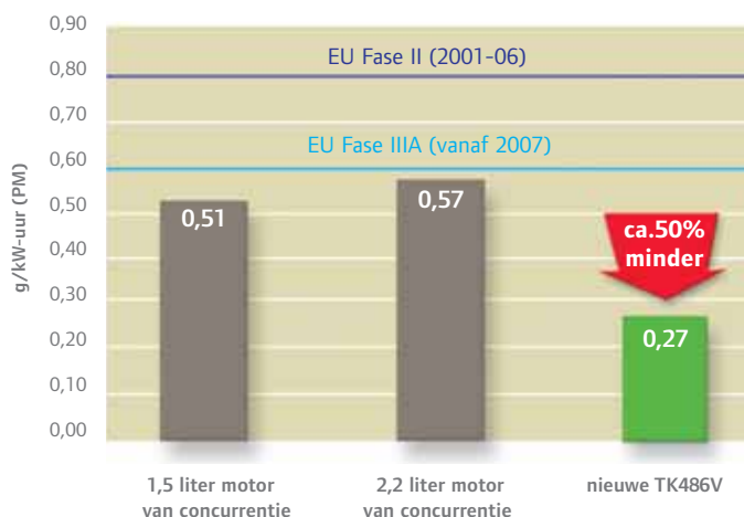
Uitstoot (van deeltjes): Concurrende motoren versus nieuwe motoren voor opleggerunit
